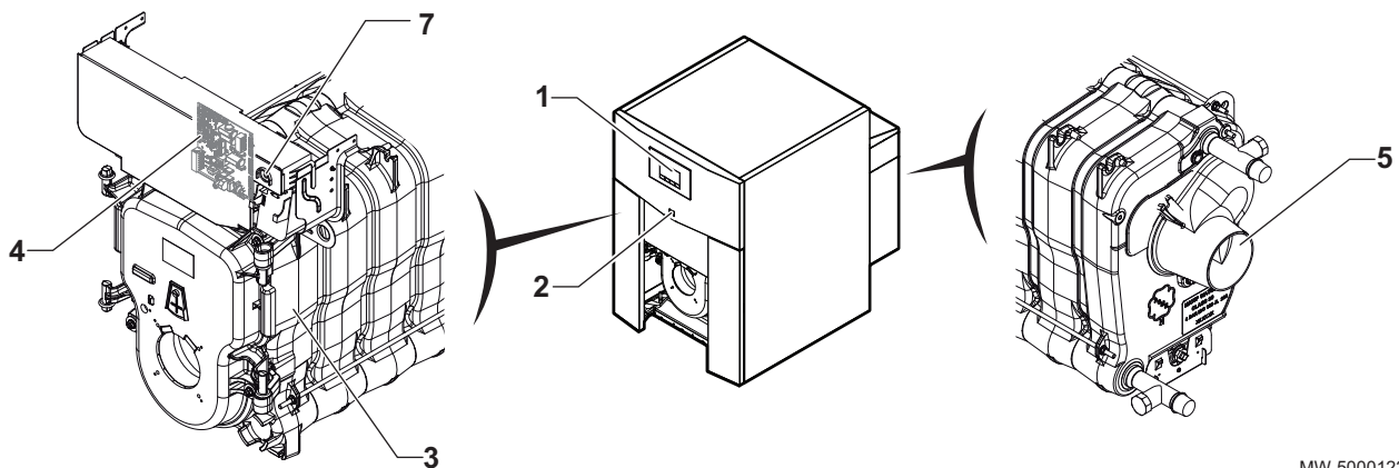
Abb.2 Hauptkomponenten
