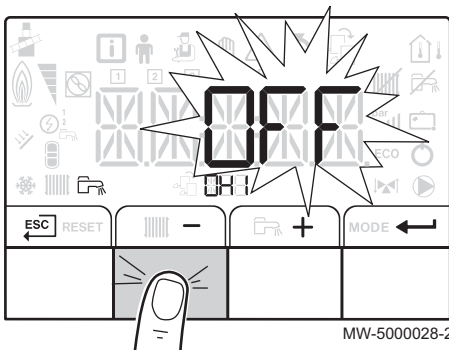
Abb.33 Warmwasserproduktion ausschalten
