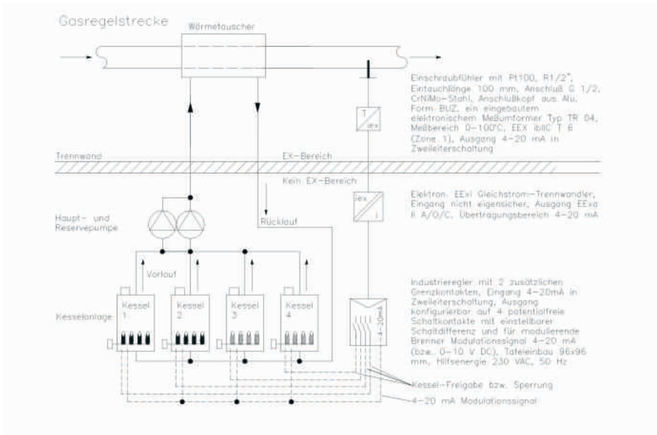
Schematischer Aufbau einer Gasregelstation mit Industrieregler und modulierenden Brennern
