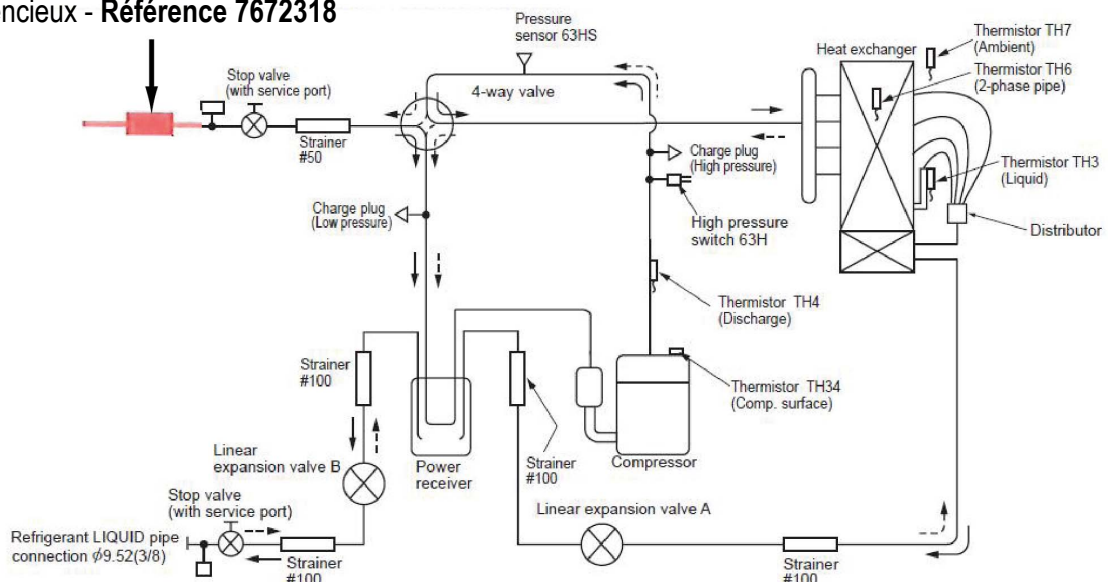
Silencieux - Référence 7672318
